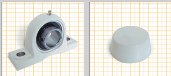
SOPORTE OMEGA CON TAPA CERRADA UCP / OMEGA SUPPORT WITH CLOSED COVER UCP PALIER A SEMELLE UCP CAPOT FERMÉ / STEHLAGER SERIE UCP MIT SCHUTZKAPPE, GESCHLOSSEN
