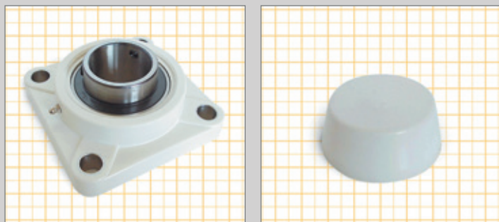
SOPORTE CUADRADO CON TAPA CERRADA UCF / SQUARE SUPPORT WITH CLOSED COVER UCF PALIER CARRÉ UCF CAPOT FERMÉ / FLANSCHLAGER 4-LOCH-BEFESTIGUNG SERIE UCF MIT SCHUTZKAPPE, GESCHLOSSEN
