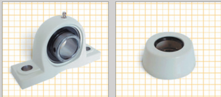
SOPORTE OMEGA CON TAPA ABIERTA UCP / OMEGA SUPPORT WITH OPEN COVER UCP PALIER A SEMELLE UCP CAPOT OUVERT / STEHLAGER SERIE UCP MIT SCHUTZKAPPE, OFFEN
