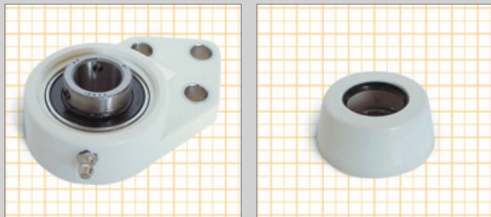
SOPORTE CABEZAL TENSOR CON TAPA ABIERTA SQL HEAD TENSILE SUPPORT WITH OPEN COVER SQL PALIER SQL STANDARD CAPOT OUVERT FLANSCHLAGER SERIE SQL MIT SCHUTZKAPPE, OFFEN
