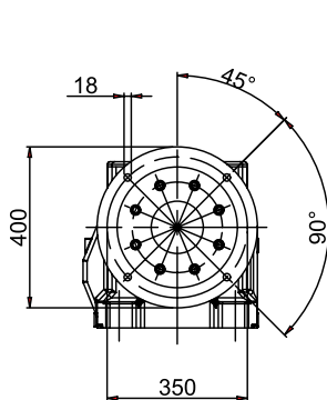
Flangia Riportata Bride modulare
