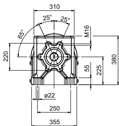
Flangia Riportata Bride modulaire
