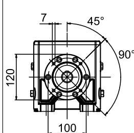
Flangia Riportata Bride modulaire
