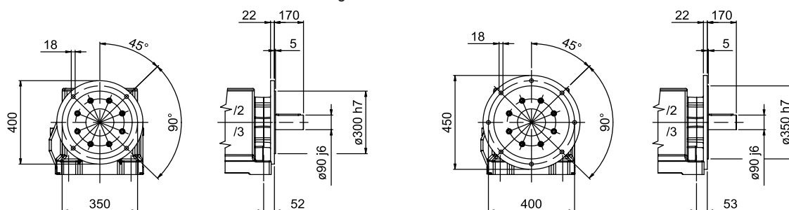
Eingebauter Flansch Flange modular
