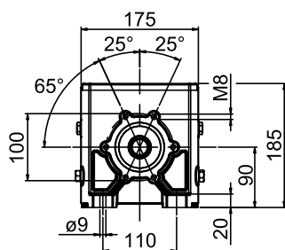
Flangia Riportata Bride modulaire
