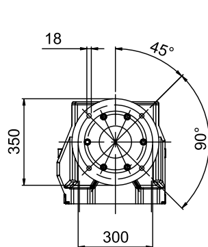
Flangia Riportata Bride modulaire
