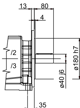
Eingebauter Flansch Flange modular
