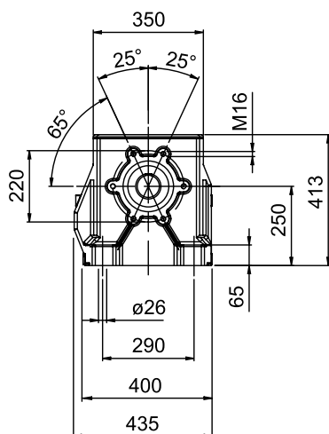
Flangia Riportata Bride modulaire
