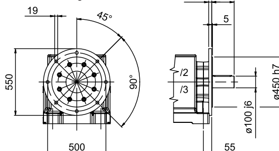
Eingebauter Flansch Flange modular
