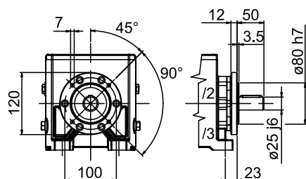
Flangia Riportata Bride modulaire
