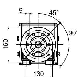
Eingebauter Flansch Flange modular
