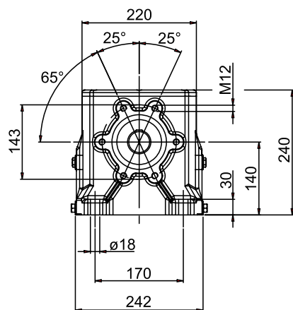
Flangia Riportata Bride modulaire
